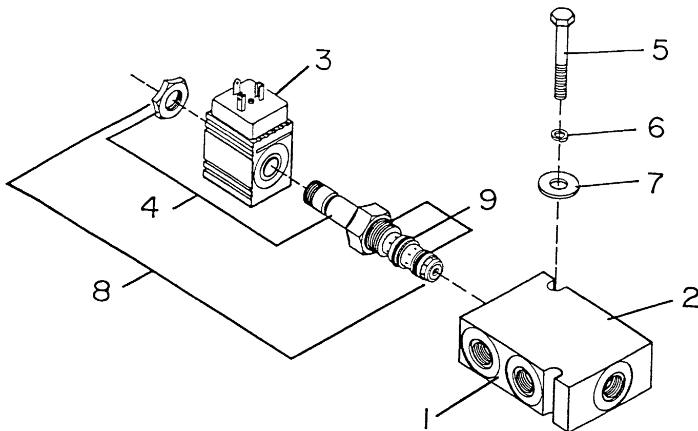
ASSEMBLY ITEMS 2,3,4
